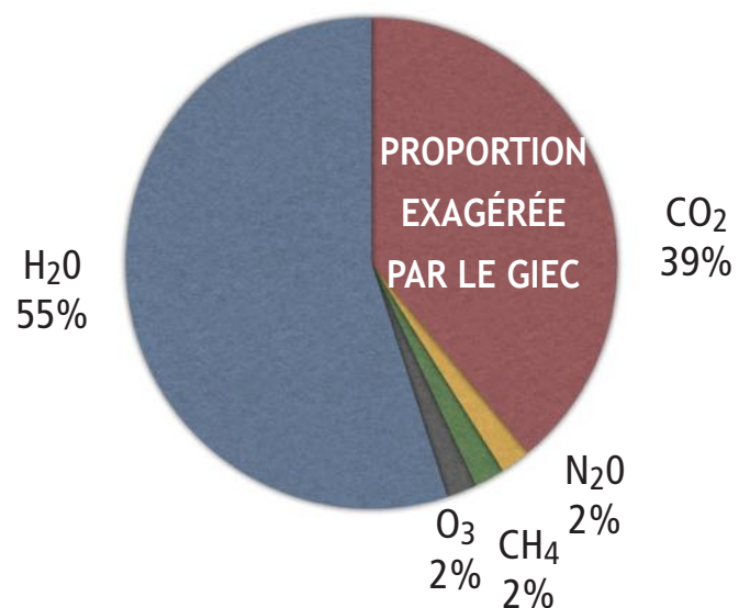
Répartition des contributions à l'effet de serre des différents gaz présents dans l'atmosphère en 1992. (selon le GIEC)
